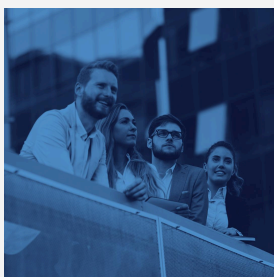
AI NAVIGATOR
